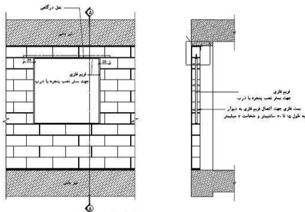
جزئیات اجرایی نصب فریم فلزی جهت بستر نصب در و پنجره
