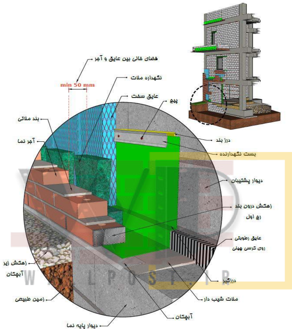
شکل پ ۶-۳۹-جزئیات اجرای نمای آجری
