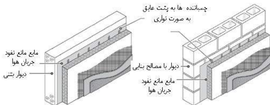
شکل پ-۲۶- نحوه صحیح اجرای نمای سیمانی مسلح شده به مش الیاف و عایق حرارتی بر روی دیوار
