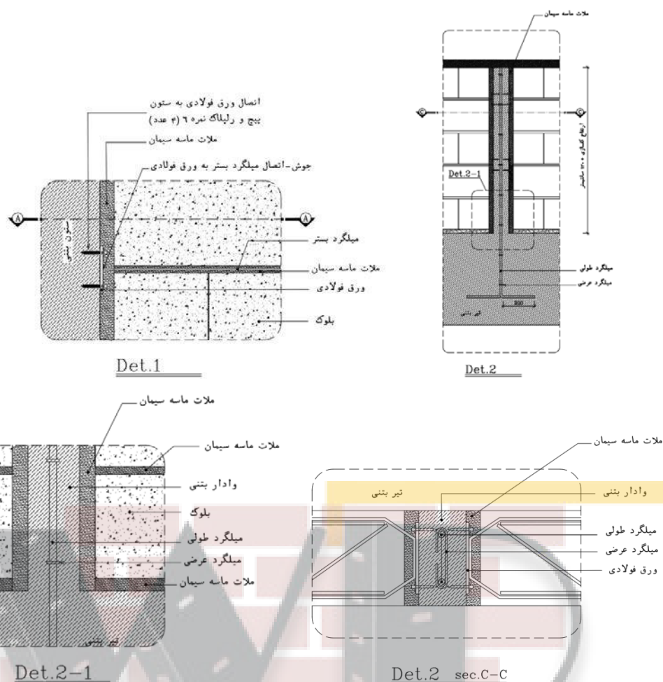
شکل پ ۶-۳۷- جزئیات اجرایی اتصال جان پناه با وادار بتنی
