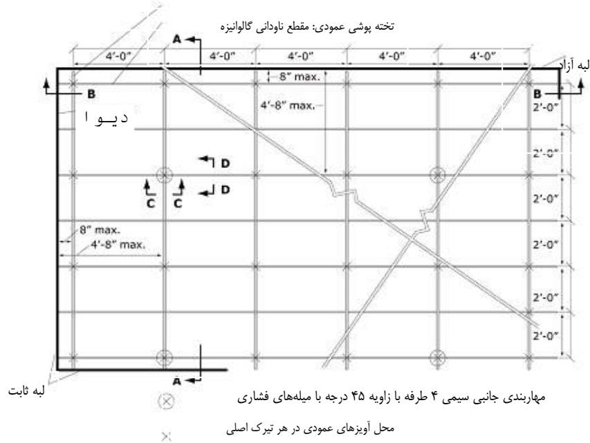
شکل پ-۳۳-۶- پلان مهاربندی عرضی برای شبکه سقف سنگین معلق (جزئیات مقاطع در شکل پ-۳۹-۶ ارائه شده است)
