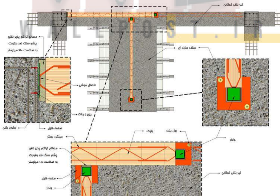
شکل پ ۶-۱۳- اجرای دیوارهای متقاطع و نحوه اجرای وادار در محل اتصال دو دیوار
