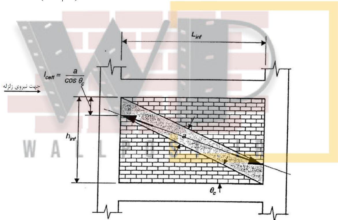
شکل پ ۶-۴۲- نیروی وارد به ستون از طرف میانقاب
