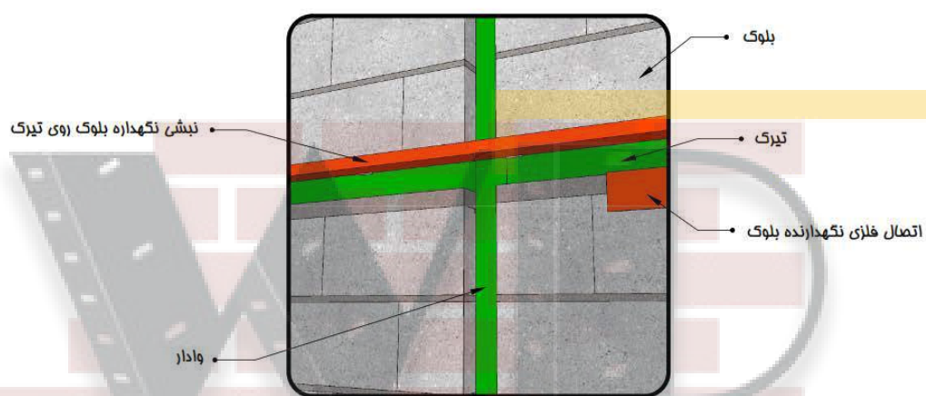
میزانیات اتصال تیرک به وادر
