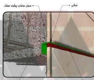
جزئیات اتصال پلی استایرن به سنگ به تور بتنی کفانی det.1
