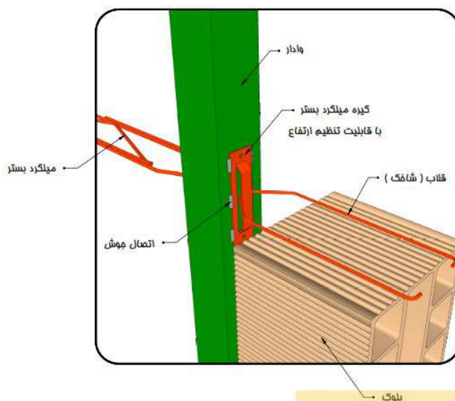
شکل پ ۵-۶- میلگرد بستر در فاصله بین وادارها و اتصال آن به وادر
