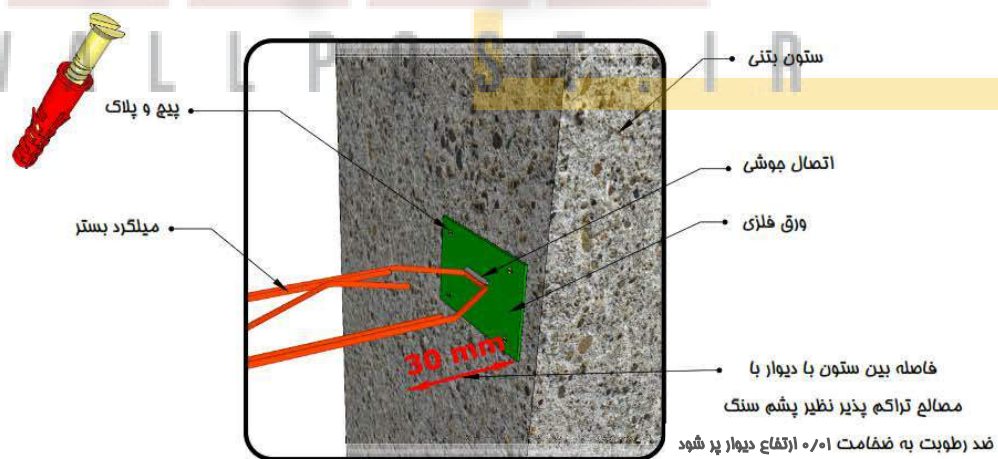
میزانیات اتصال میلگرد بستر به ستون بتنی
