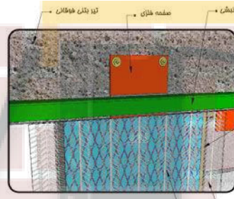
جزئیات استقرار رابکس و پلی استایرن روی ستون بتنی det.2
