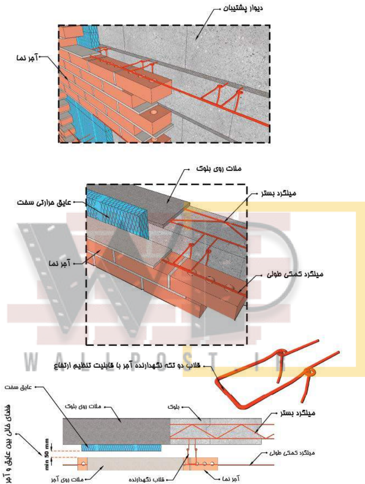
شکل پ ۶-۲۸- نحوه مهار نمای آجری به دیوار پشت
