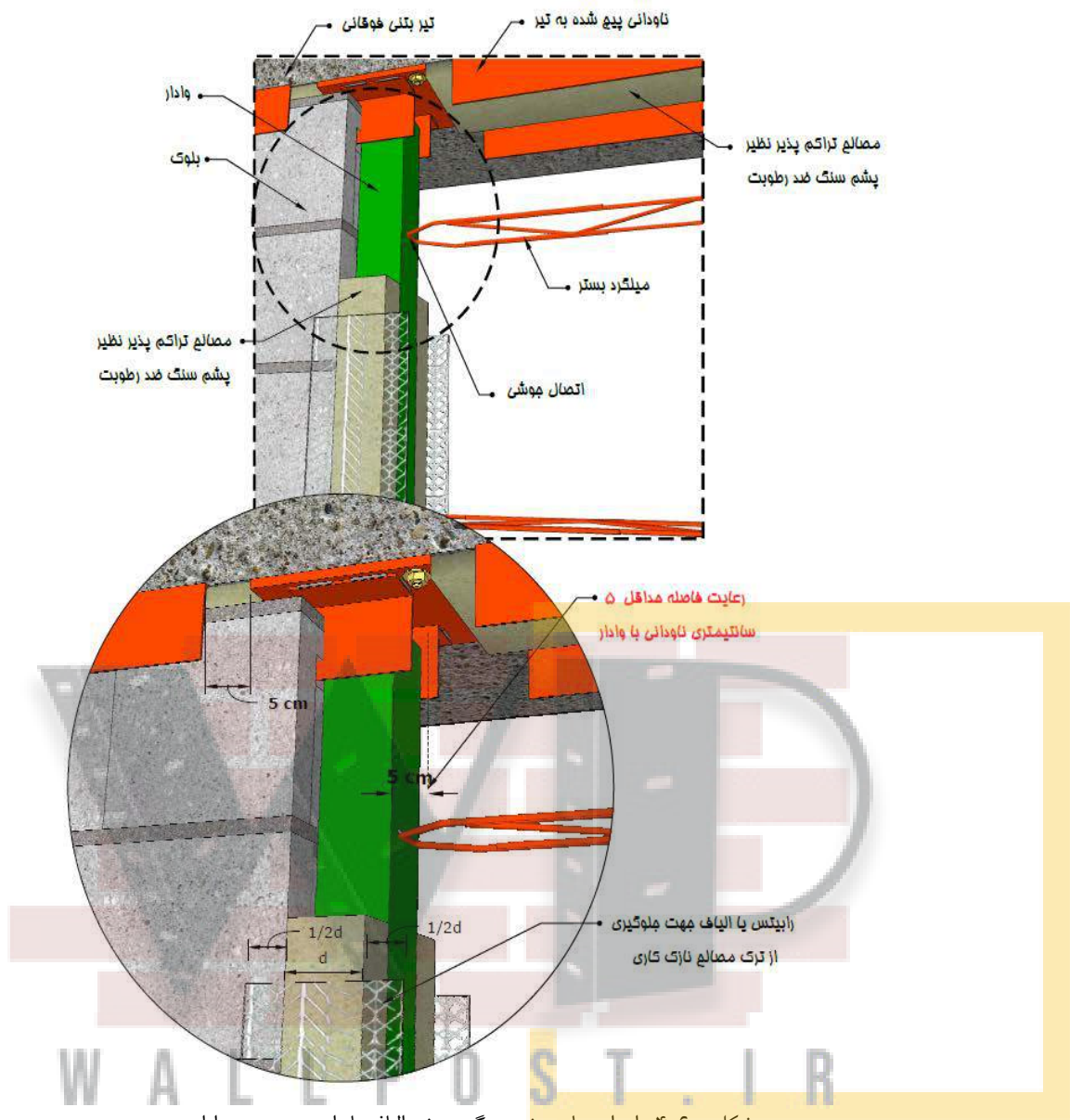
شکل پ ۴-۳-۱- اتصال به وادارها
