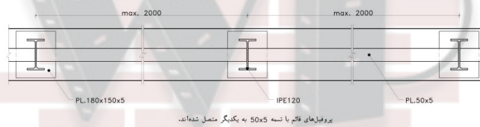
SEC. a-a
