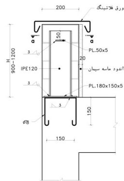
جزئیات جان پناه یا مصالح بنائی
