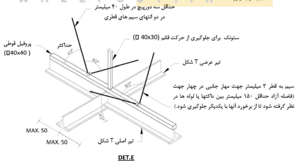
DET. E
