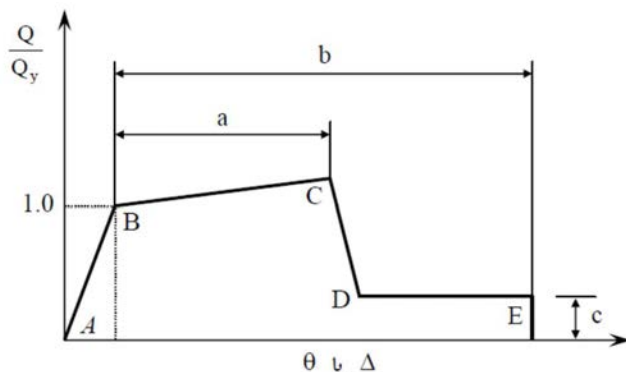
شکل ۲-۱- منحنی ساده شده نیرو-تغییر شکل اعضاء
