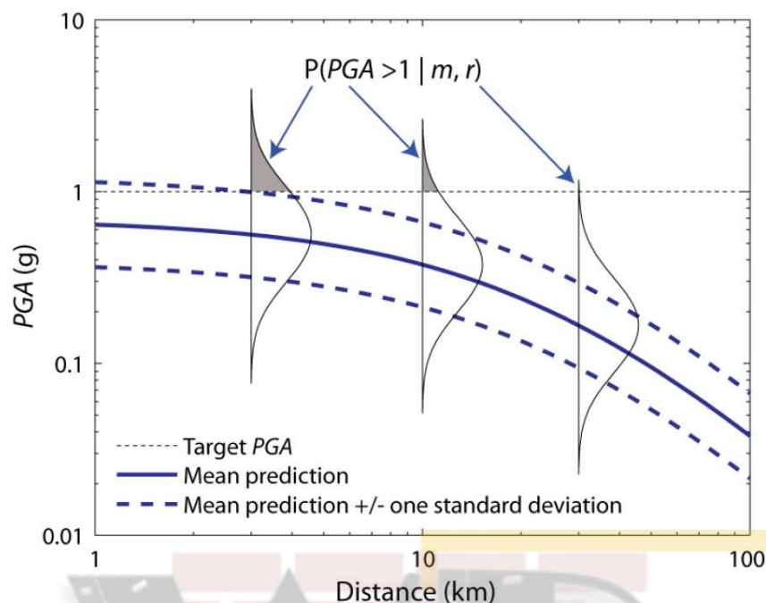
شکل ۴-۱۹- نحوه اعمال عدم قطعیت توابع کاهندگی در فرآیند تجميع احتمالات خطر زلزله Baker, 2008
