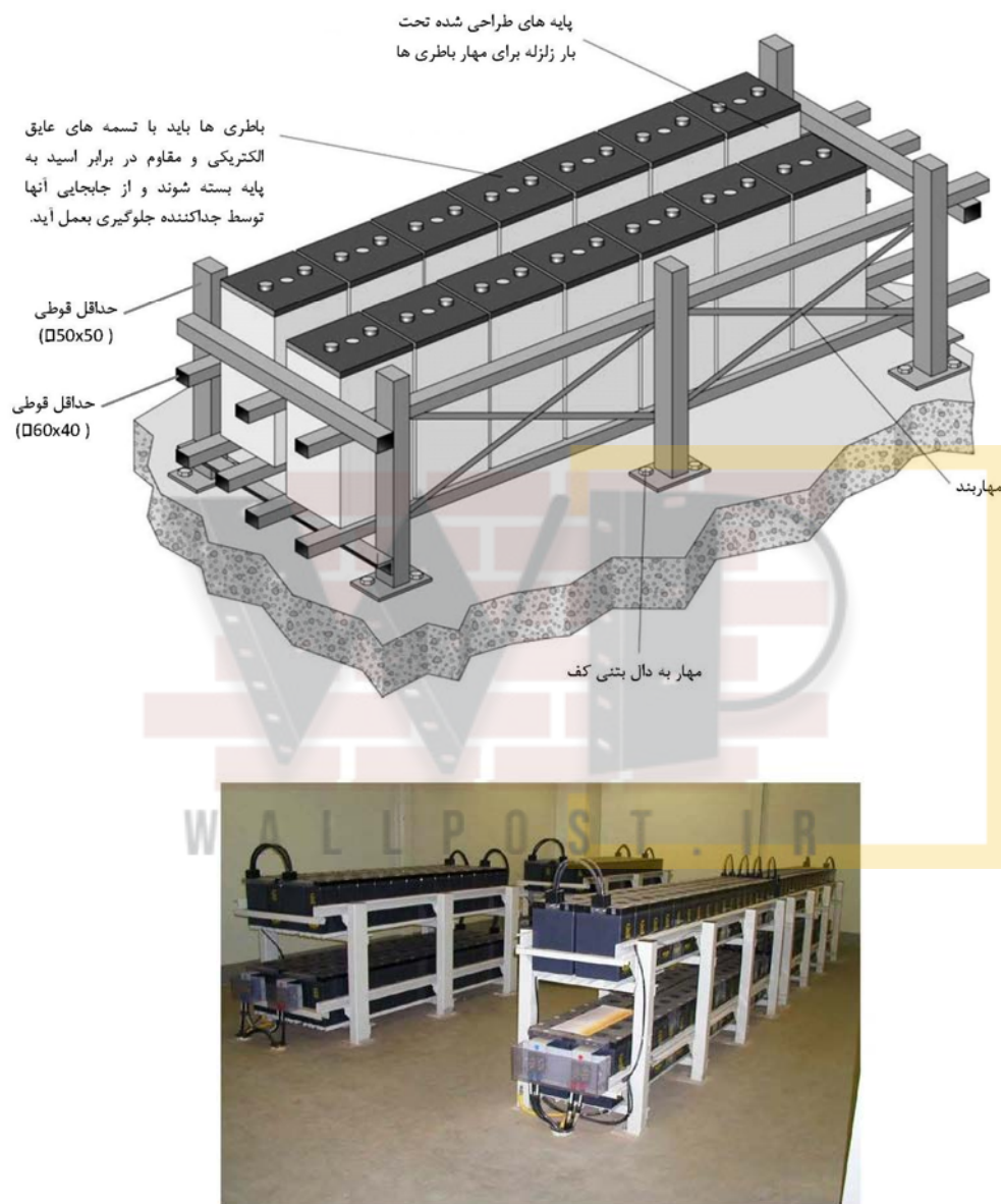
شکل ۳-۲۵- جزئیات مهار باطری ها
