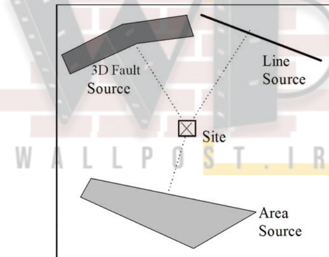
شکل ۴-۱- مدل‌های هندسی قابل استفاده برای مدل‌سازی منابع لرزه‌ای
