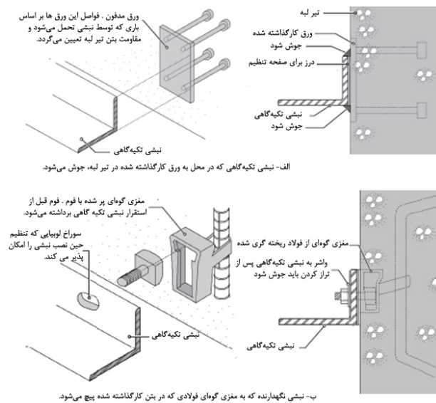
شکل ۵-۲۰- جزئیات اجرایی اتصال نشی تکیه‌گاهی به دیوار پشتیبان
