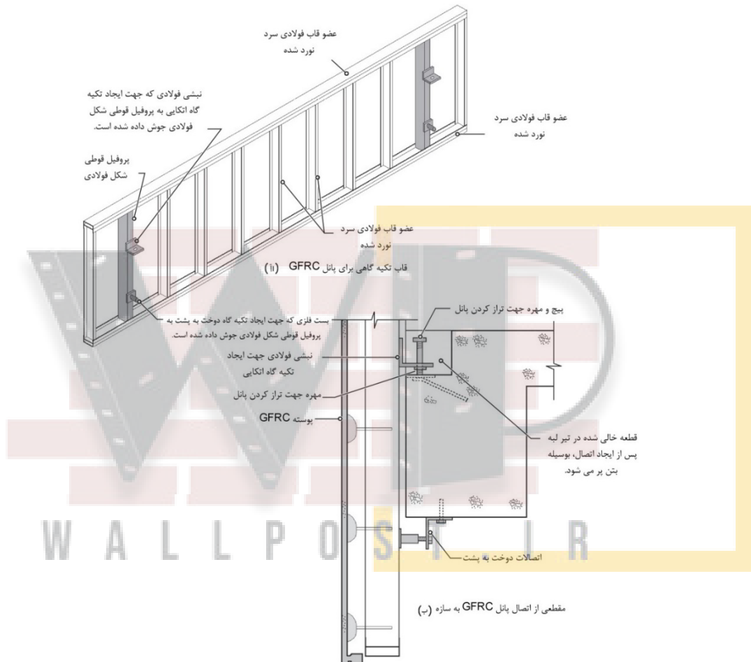
شکل ۱۱-۱۶- تصویری شماتیک از جزئیات اتصالات اتکایی و دوخت به پشت در پانل‌های پیرامونی GFRC
