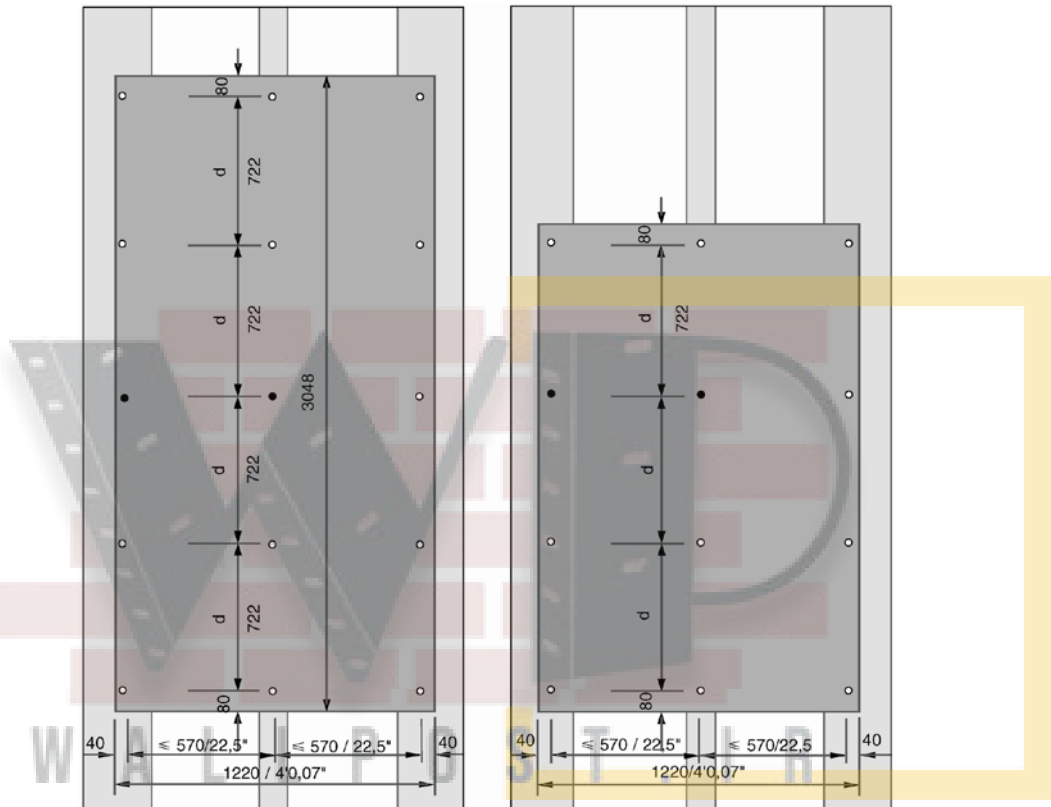
شکل ۱۱-۲۲- نمونه جانمایی و تعیین محل‌های نصب صفحه سیمانی بر روی زیرقاب
