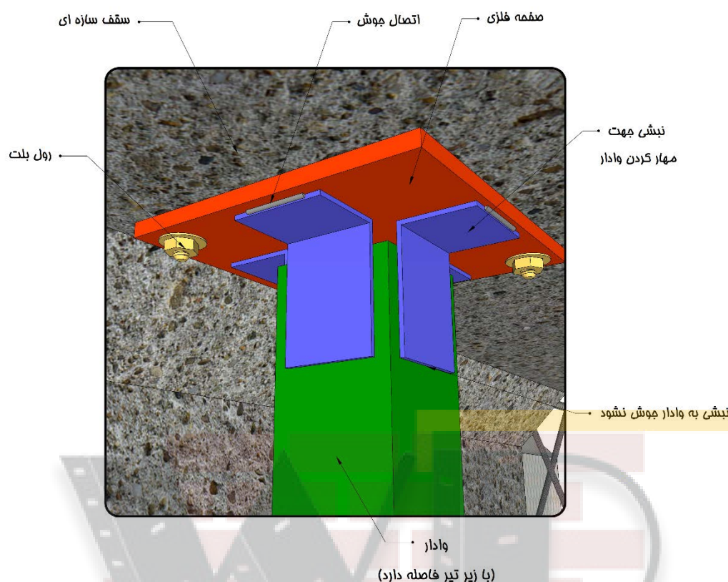
ب- اتصال وادار انتهایی در دیوارهای خارج از قاب به صورت تلسکوپی شکل ۱۲-۹- اتصال وادار به سقف
