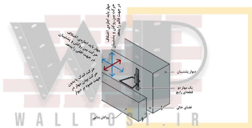
شکل ۵-۶- تنظیم‌شوندگی مورد نیاز در جهت‌های مختلف مهر دو تکه
