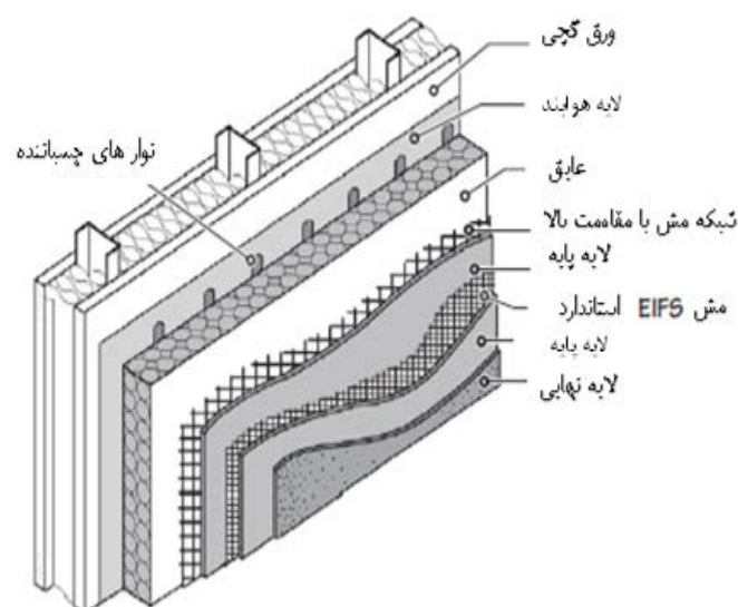
شکل ۱۱-۹ جزئیات نمای EIFS مقاوم در برابر ضربه که شامل دو شبکه ایاف است
