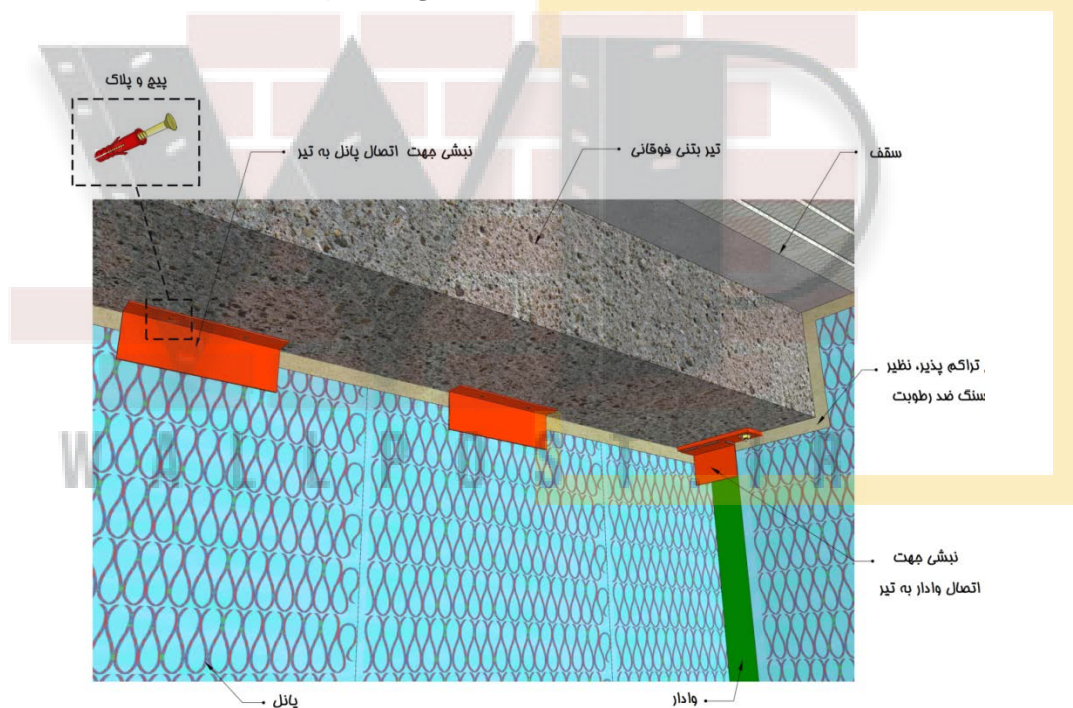
شکل ۱۲-۳۱- جزئیات نحوه مهار دیوار پانلی نیمه پیش ساخته در سقف طبقات
