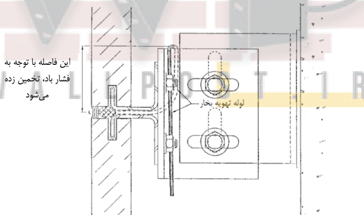
شکل ۴-۲۲- لوله تهویه بخار
