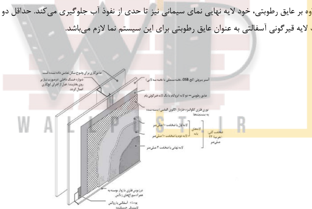
شکل ۶-۱ ساختار اجرای نمای سیمانی روی دیوار خشک
