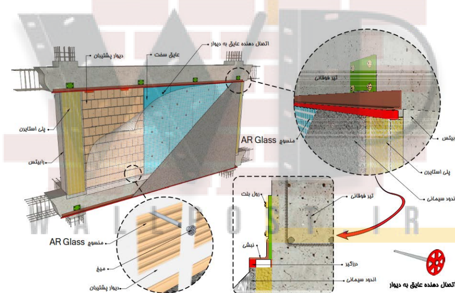
شکل ۱۱-۲۰- نمای بتن مسلح شده با منسوج (شبكة الیاف) در دیوارهای نیازمند به عایق حرارتی مانند سفال
