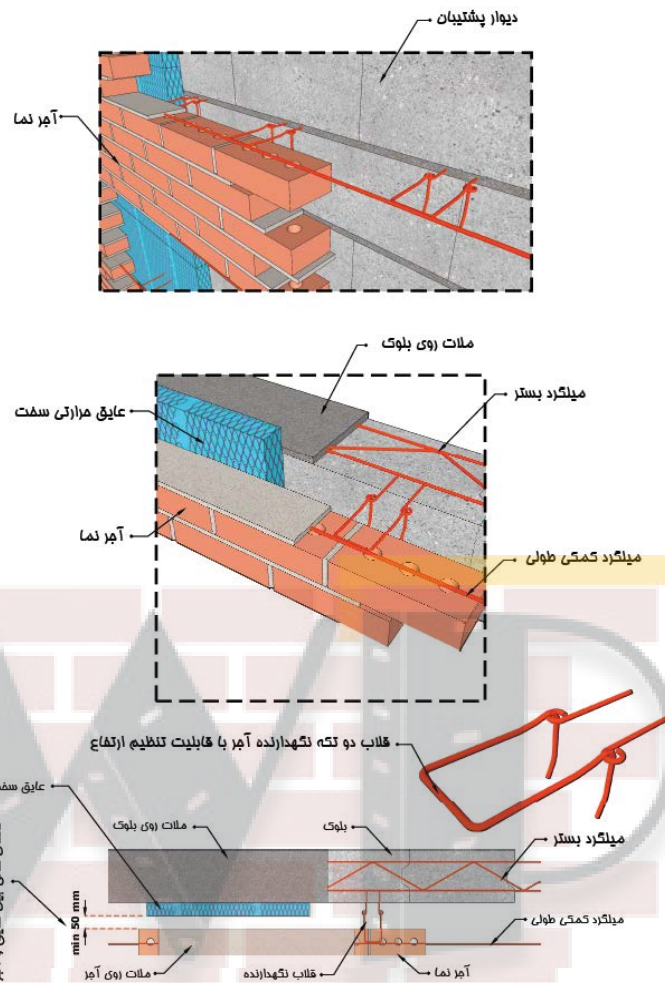
شکل ۵-۱۹- نمای آجری متصل به دیوار پشتیبان
