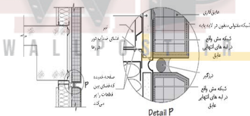
شکل ۱۱-۸- جزییات درزهای لرزه‌ای و انبساطی در دیوار نما EIFS
