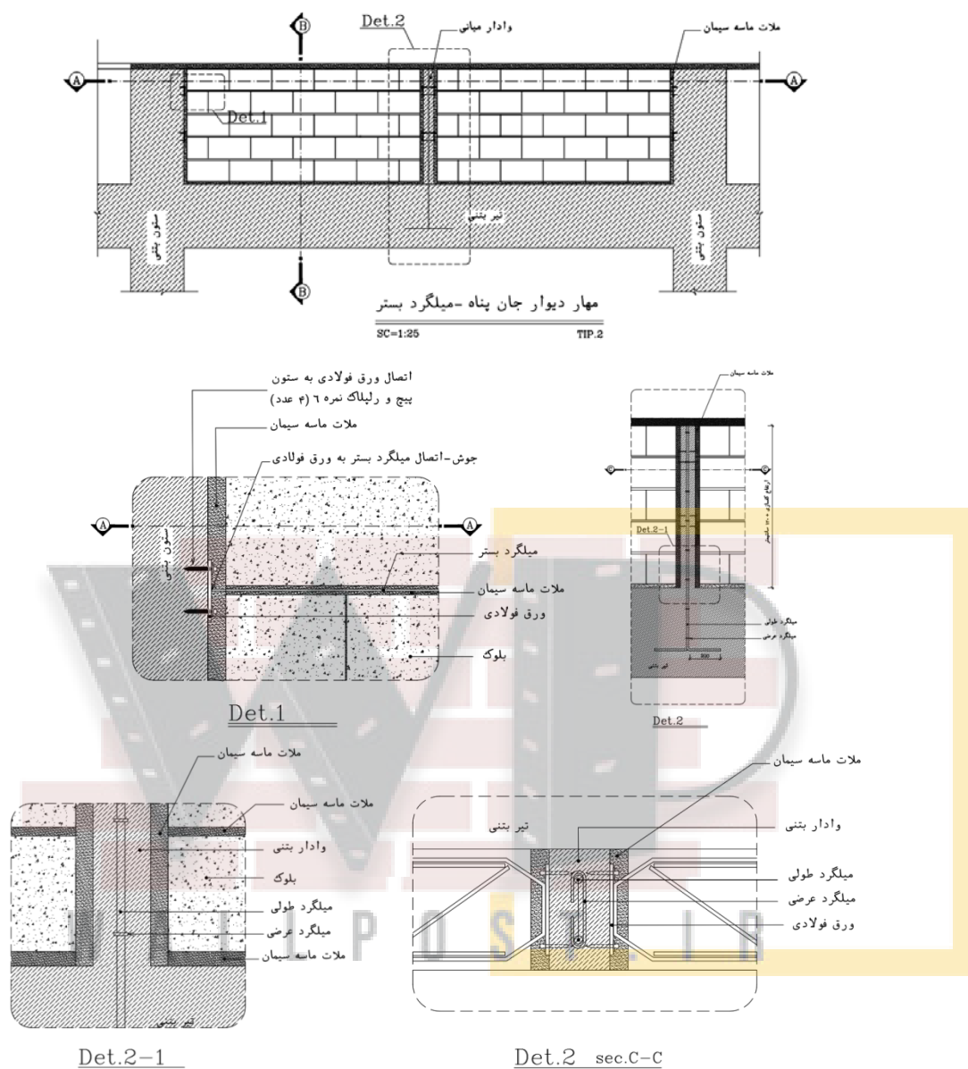
شکل ۱۲-۳۴- جزئیات اجرایی اتصال جان پناه با وادار بتنی
