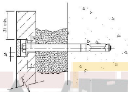
شکل ۴-۳- مهاری سطحی
