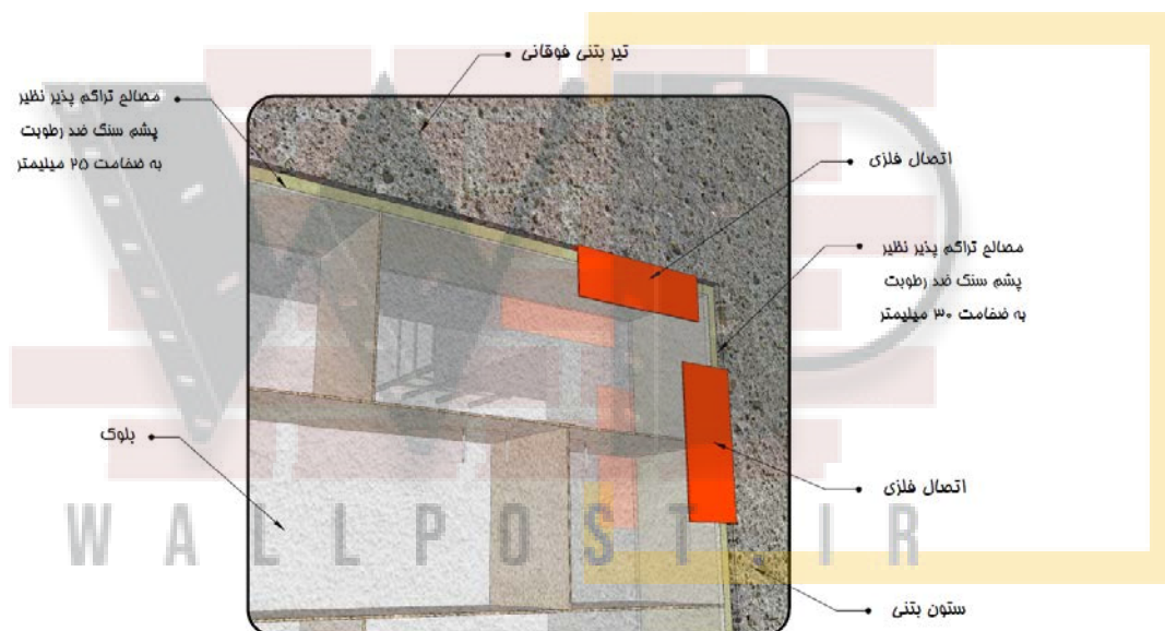
شکل ۱۲-۱۵- جزئیات اجرایی در محل تلاقی دیوار با سقف - اتصال دیوار به سقف با استفاده از نبشی
