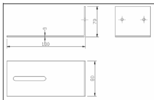
شکل ۷-۲-۷- براکت‌ها (نشیمن‌های) گوشه
