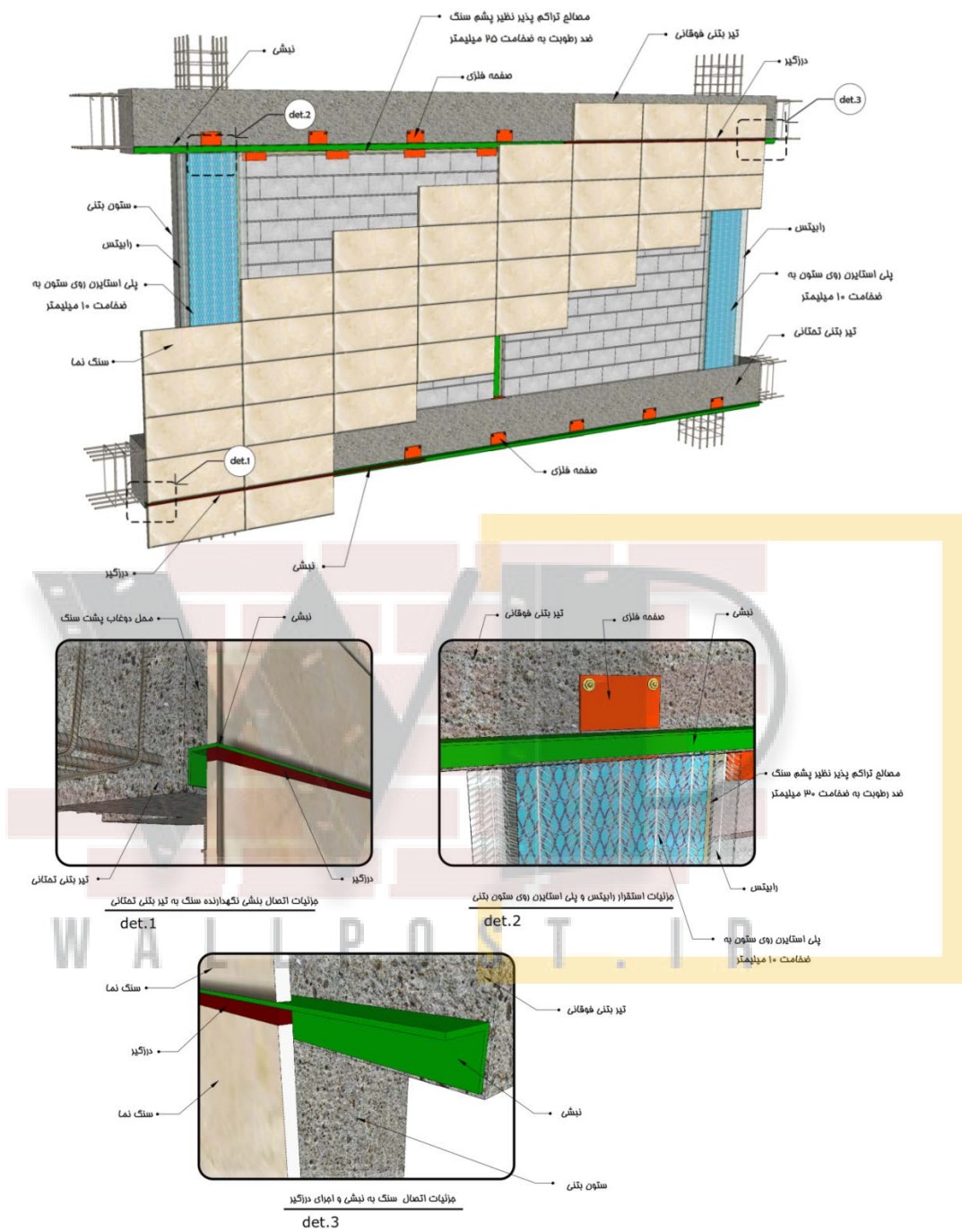
شکل ۴-۱۹- نحوه اجرای نمای چسبانده شده در دیوارهای جداسازی شده
