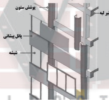
شکل ۹-۵- سیستم نمای پرده‌ای پوشش ستون و تیر پیشانی
