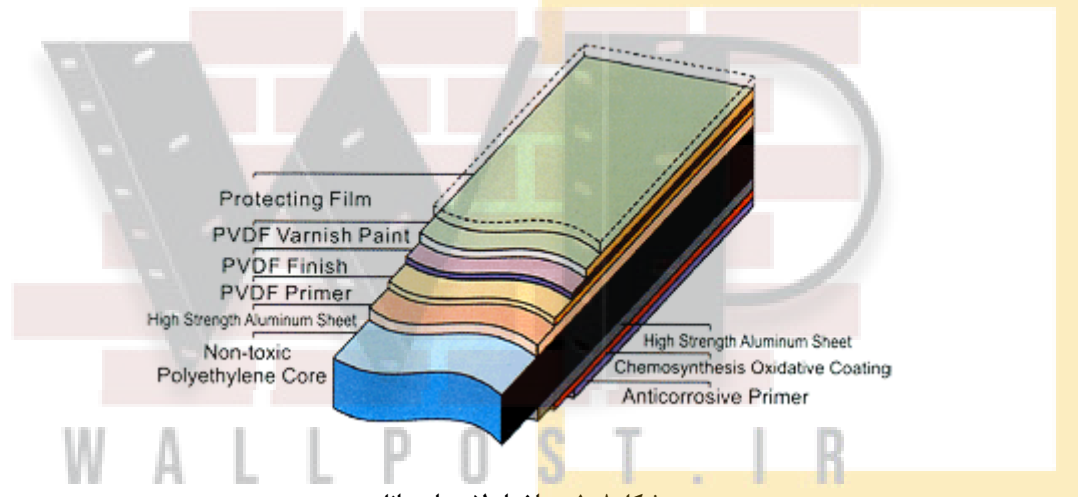
شکل ۸-۱- ساختار لایه‌های پانل
