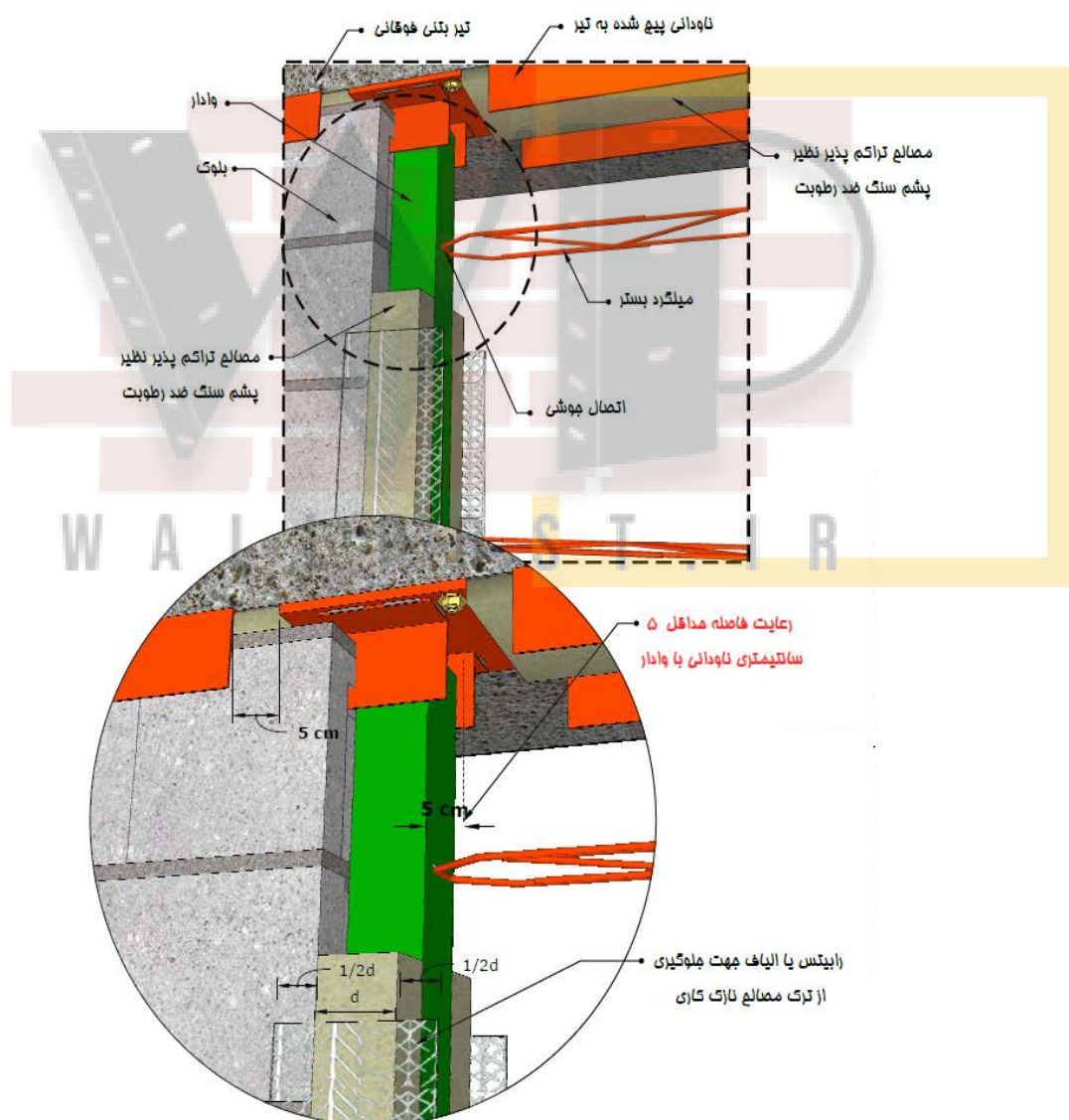
شکل ۱۲-۷- اجرای عایق پشم سنگ و مش الیاف یا رابیتس بر روی وادار
