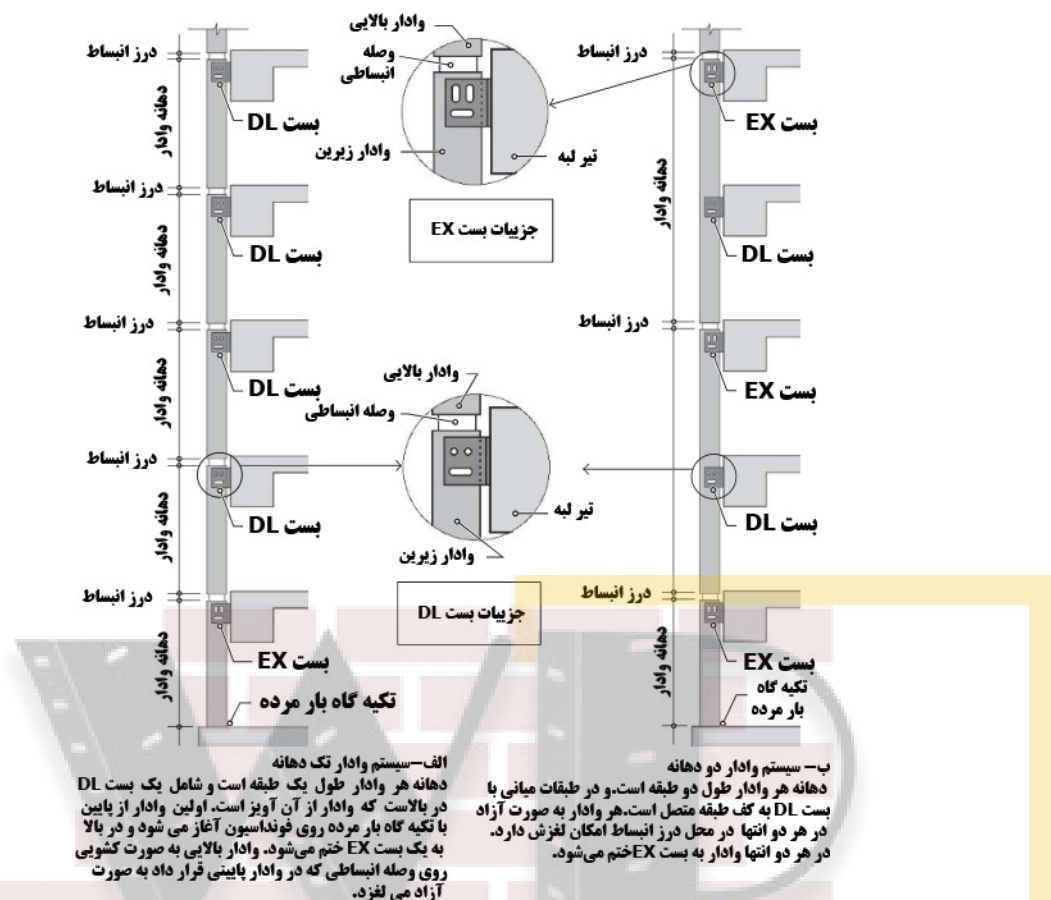
شکل ۹-۸- سیستم های تکیه گاهی برای دیوارهای پرده ای شیشه با وادار تک و دو دهانه
