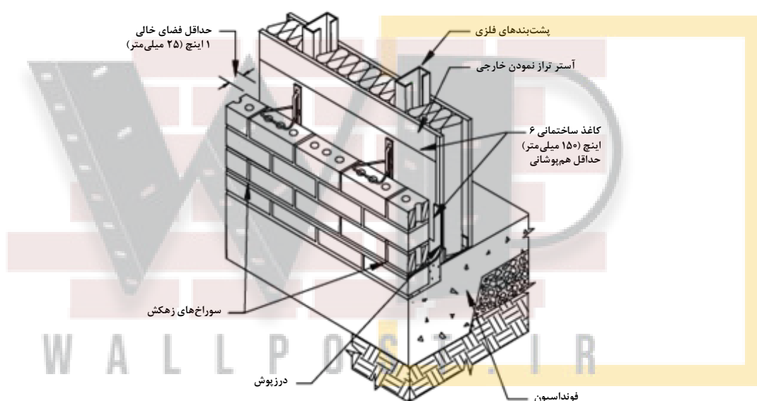
شکل ۵-۳- نمای مهاری
