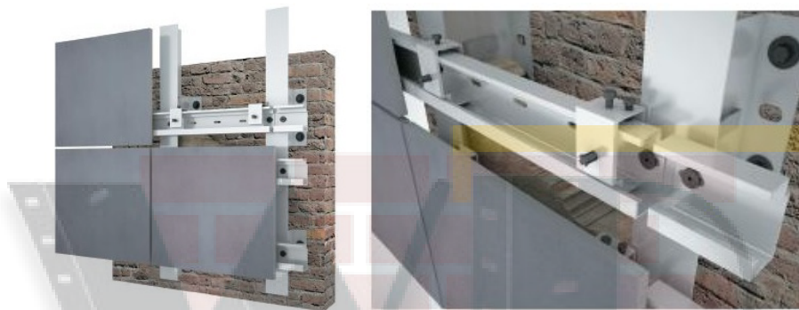
شکل ۷-۱۲- سیستم نصب پنهان با ایجاد مهار در پشت سرامیک
