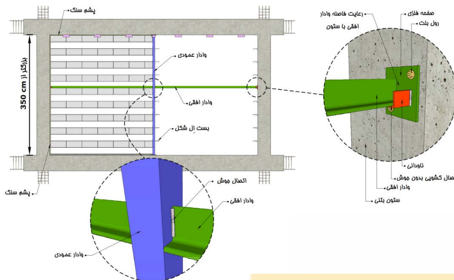
شکل ۱۰-۱۲- دیوارهای بلوکی با ارتفاع بیش از ۳/۵ متر دارای تیرک و وادر
