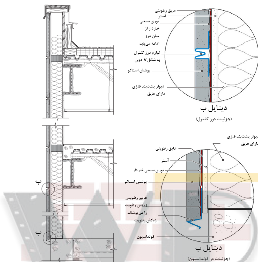
شکل ۴-۶ - یک نمونه مقطع دیوار و جزئیات متناظر از یک ساختمان قاب فلزی پوشانده شده با نمای سیمانی
