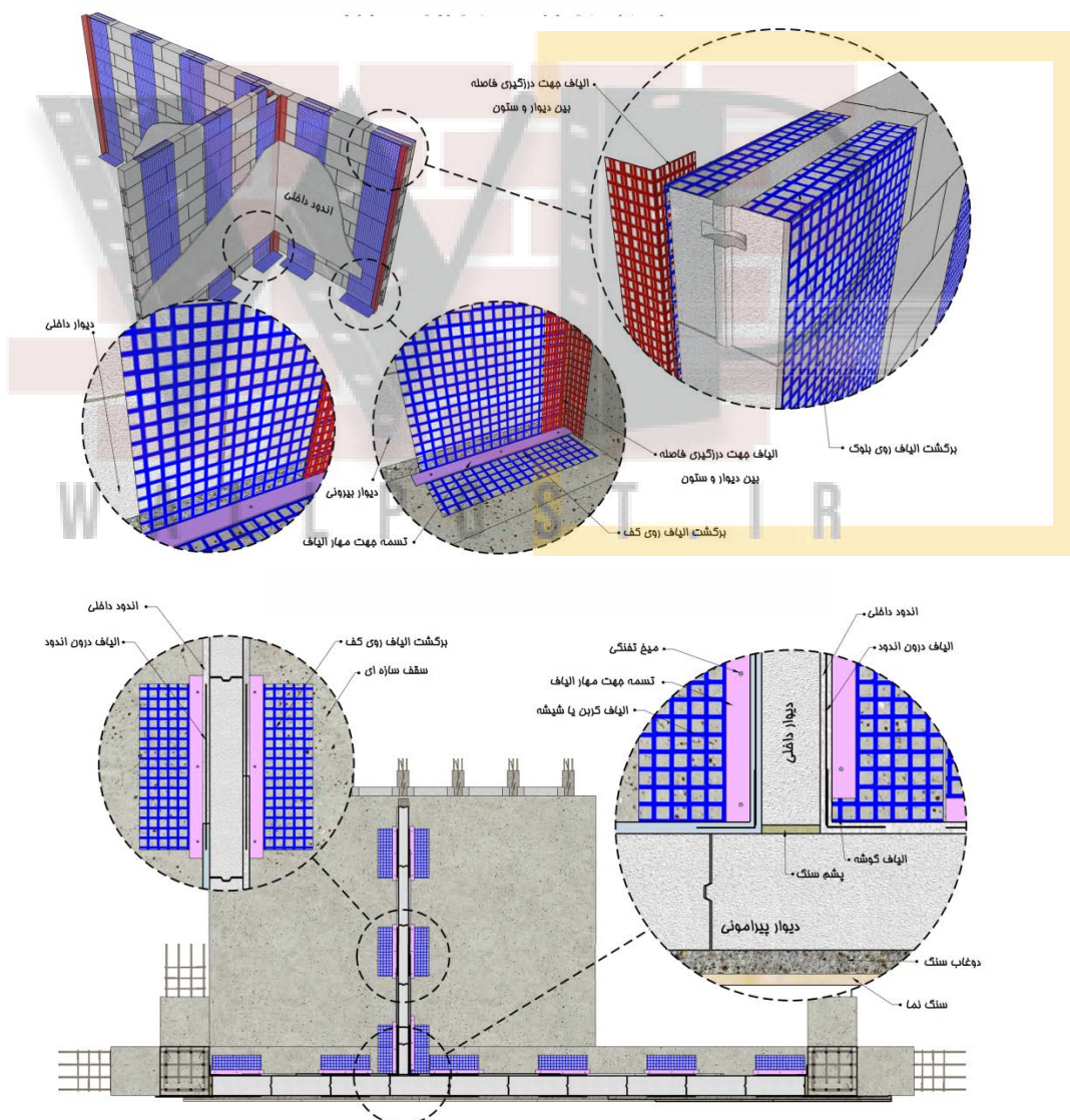
شکل ۱۲-۲۳- نحوه اجرا و تسلیح دیوارهای متقاطع با استفاده از مش الیاف
