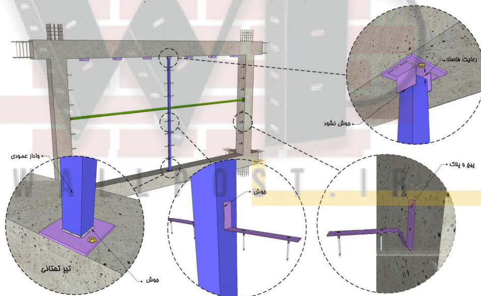
شکل ۱۱-۱۲- جزییات اجرایی اتصال تیرک و وادر در دیوار با ارتفاع بیش از ۳/۵ متر
