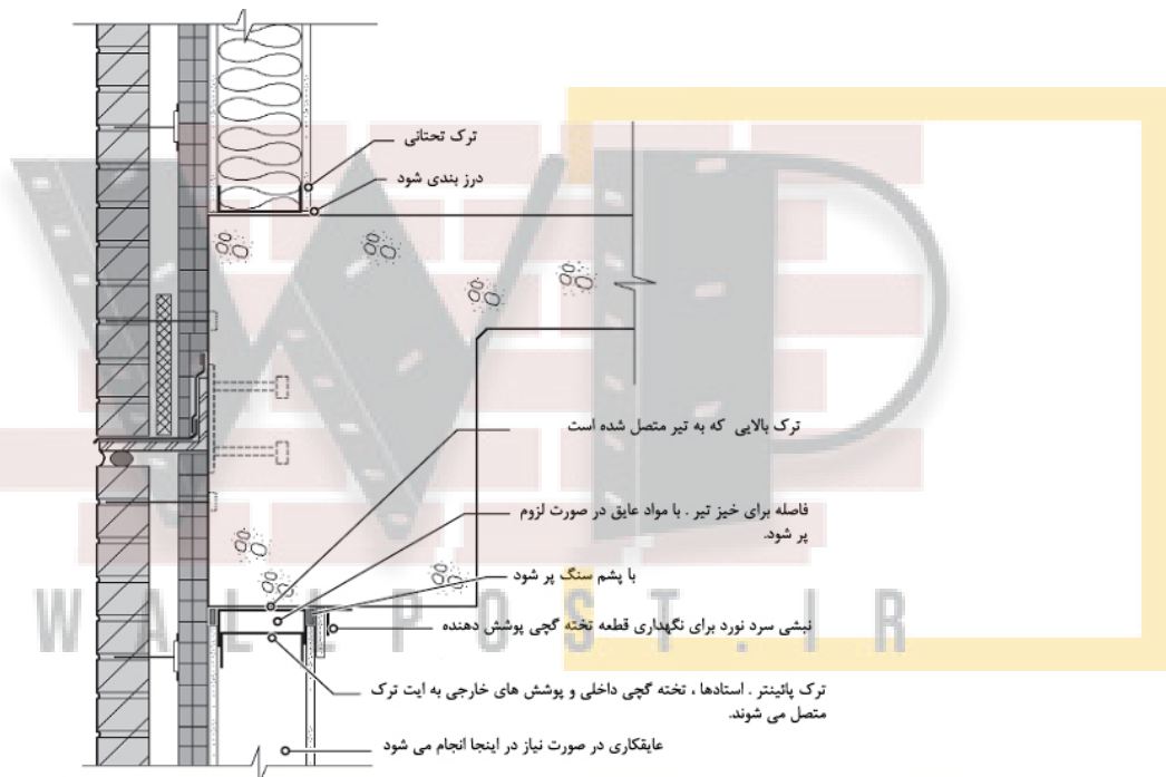
شکل ۵-۲۵- جزئیات اجرای نمای آجری بر روی پشت‌بندهای قائم فولادی، در سازه بتن آرمه
