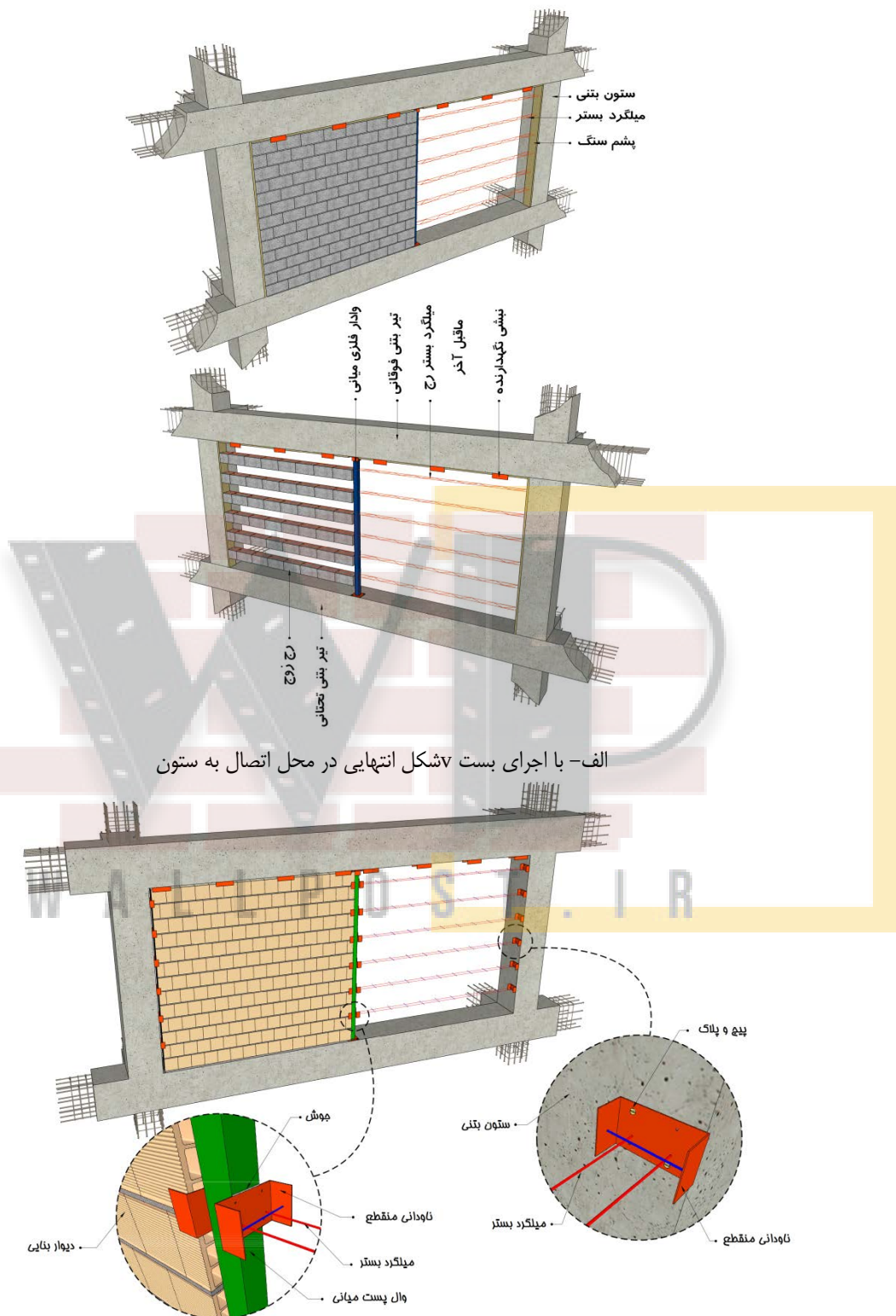
شکل ۱۲-۴- دیوار خارجی بلوکی دارای ملات سیمانی مسلح شده به میلگرد بستر
