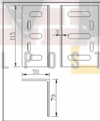
شکل ۷-۱-۷- براکت‌ها (نشیمن‌های) استاندارد
