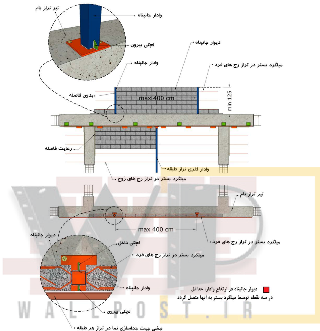
شکل ۱۲-۳۳- مهار جان پناه بنائی توسط وادر فلزی
