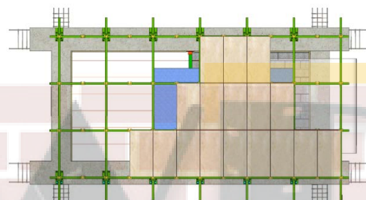
شکل ۴-۱۳- جزئیات اجرای نمای پرده‌ای سنگی
