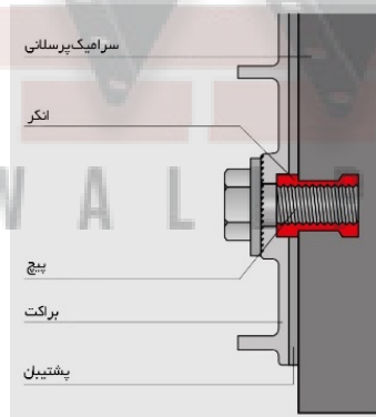
شکل ۷-۱۳- ساختار سیستم نصب پنهان به روش مهار و قلاب
