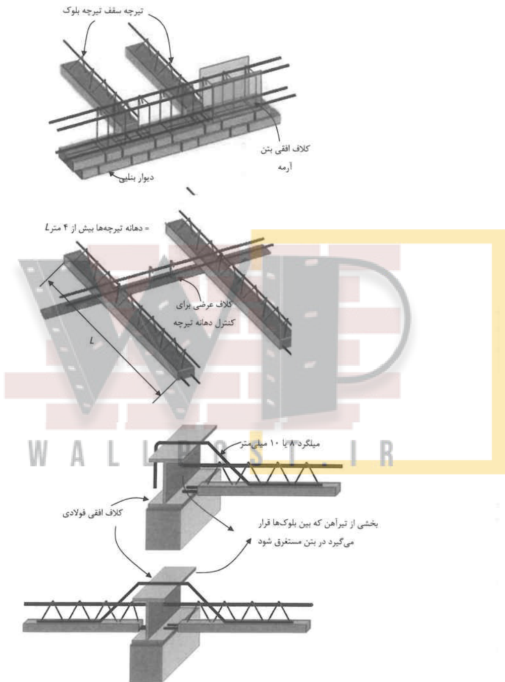
شکل ۷-۲۹ نحوه اتصال تیرچه‌های سقف به کلاف افقی بتنی و فولادی
