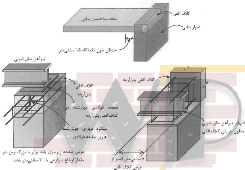
شکل ۲۶-۷ نمونه‌های اتصال تیرآهن سقف طاق ضربی به کلاف افقی بتن آرمه
