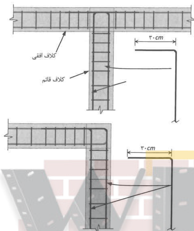
شکل ۲۱-۷ جزئیات مهار کردن میلگرد اصلی کلاف قائم در کلاف افقی
