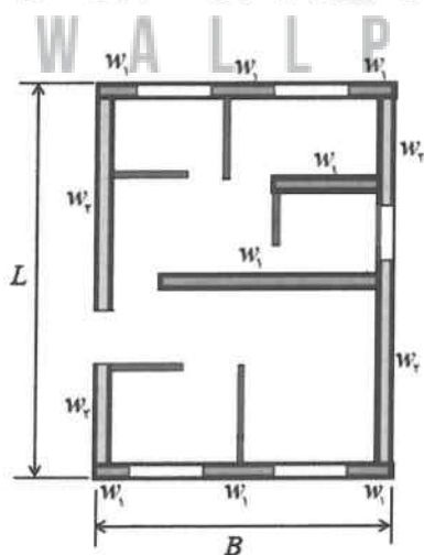
شکل ۷-۱۲ نحوه محاسبه مقدار دیوارهای سازه‌ای در هر امتداد
