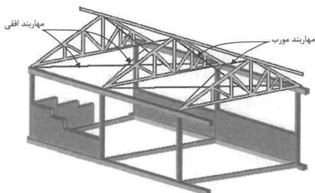
شکل ۷-۳۰ تعبیه مهاربندهای قائم و افقی در خراباها
