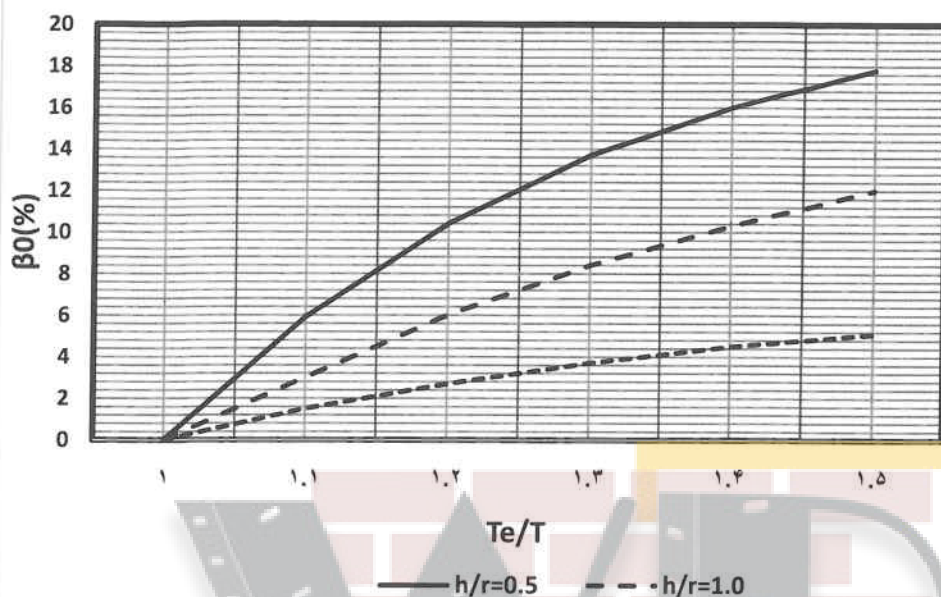
شکل پ-۵-۱ نسبت میرایی پی
