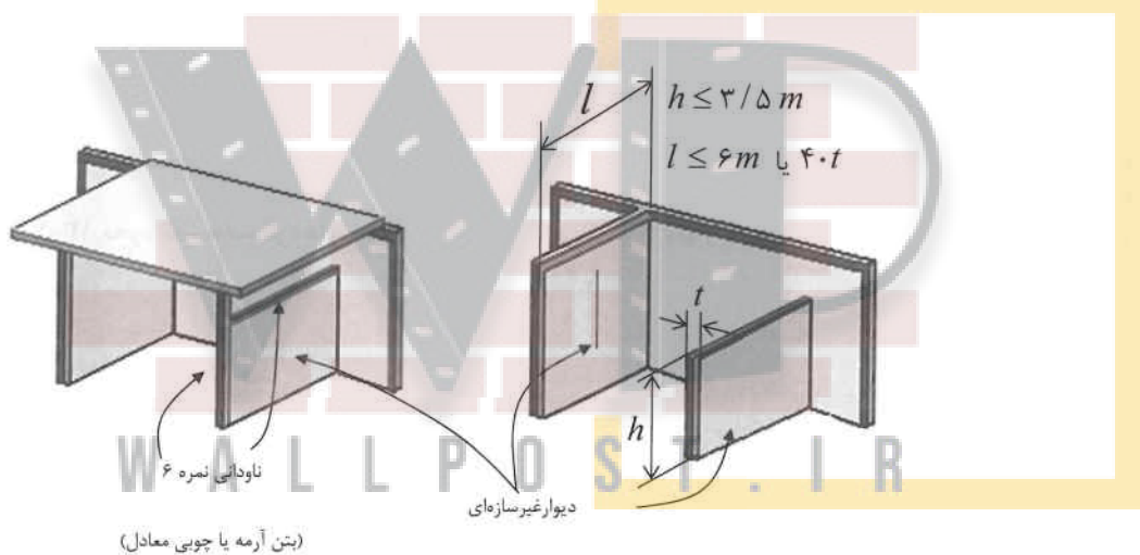
شکل ۷-۱۴ جزئیات دیوارهای غیر سازه‌ای
