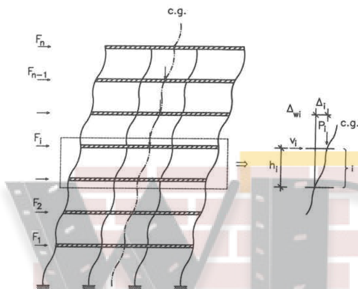
شکل پ-۳-۲ تغییر شکل‌های جانبی در اثر وارد شدن نیروهای جانبی
