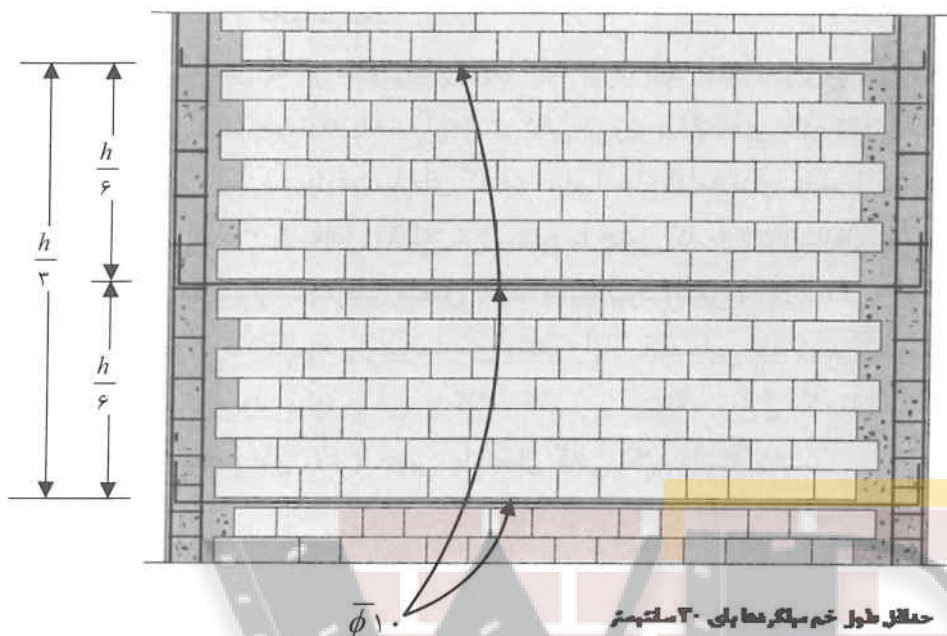
شکل ۱۳-۷ نحوه تعبیه میلگردهای ناحیه یک سوم میانی ارتفاع دیوار ( h ) و اتصال به کلاف قائم
