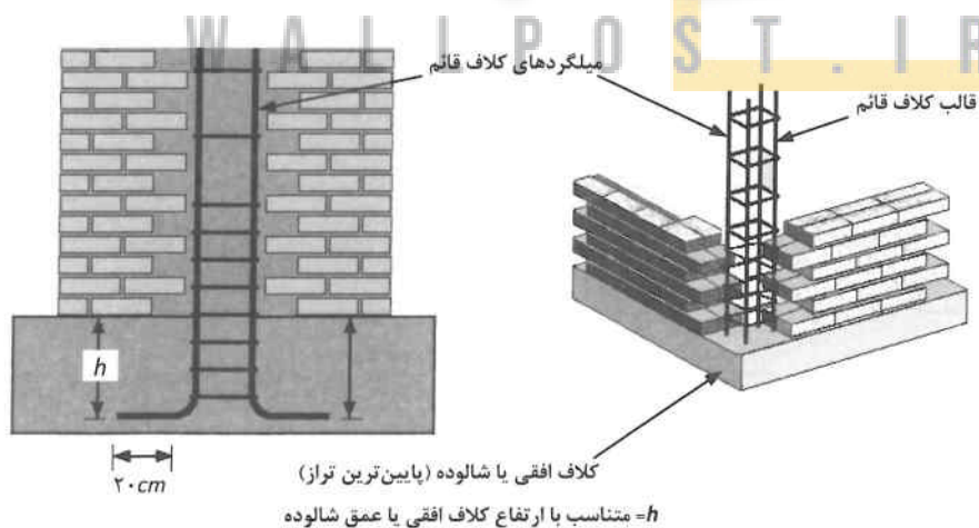
شکل ۲۲-۷ مهار میلگرد کلاف قائم در کلاف افقی یا شالوده
