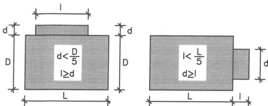
شکل ۲-۷ ابعاد پیش‌آمدگی در پلان ساختمان
